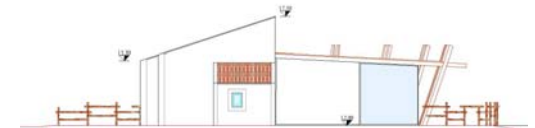
OPERE A TERRA: SEZIONI TIPO
